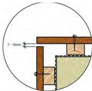
TEKENING B
