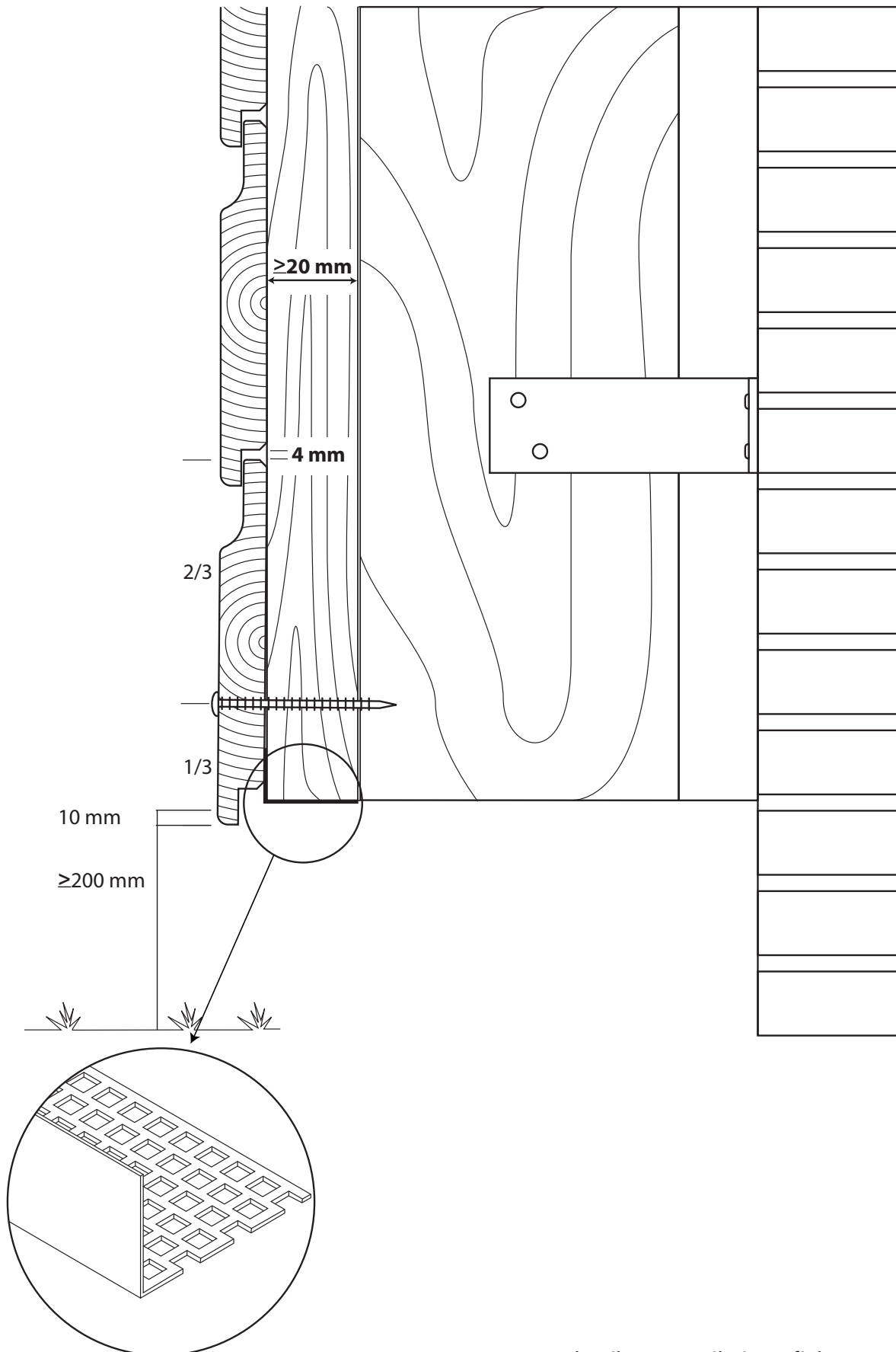
Montage detail met ventilatieprofiel
